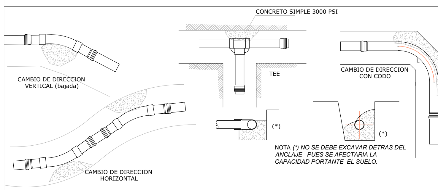
ANCLAJE DE ACCESORIOS DE TUBERIA DE ACUEDUCTO
